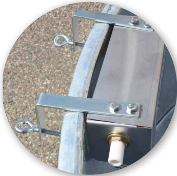
Befestigung Schwimmerkasten
