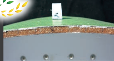
Isolierung aus Polyurethanschaum (10 mm) zwischen zwei Polyester-schichten
