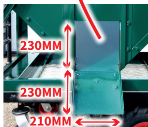
Verteilungsauslauf
