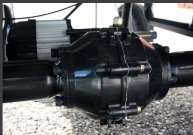
350 W-Motor mit Verteilergetriebe (2-Rad-Antrieb)
