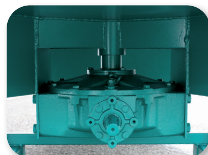
Getriebe mit Umlenkvorrichtung
